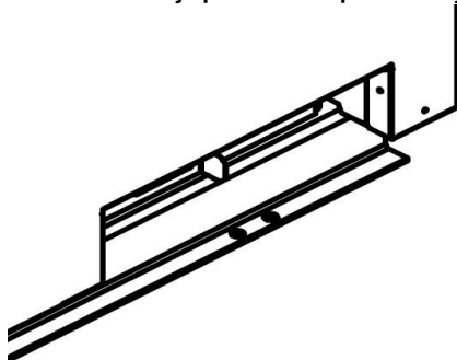
Rysunek 10. Lokalizacja przesłon doprowadzających powietrze wtórne
