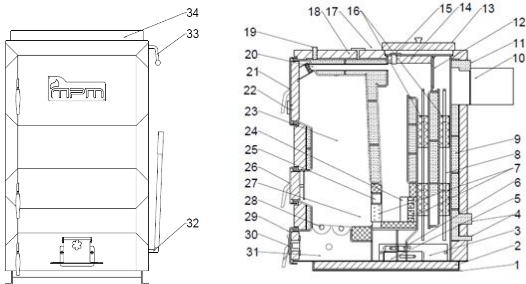
Rysunek 1. Schemat konstrukcji kotła z załadunkiem bocznym
