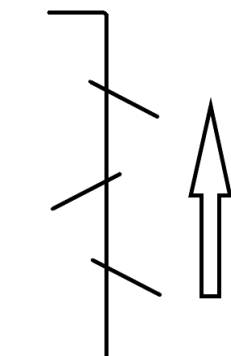
Rysunek 7. Montaż zawirowywacza w trzecim kanale spalinowym.
