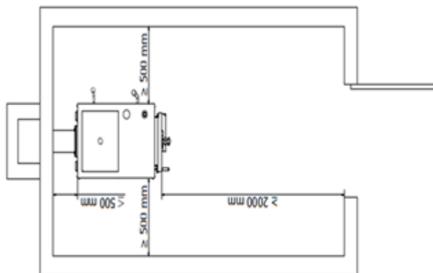
Rysunek 5. Ustawienie kotła w pomieszczeniu kotłowni.
