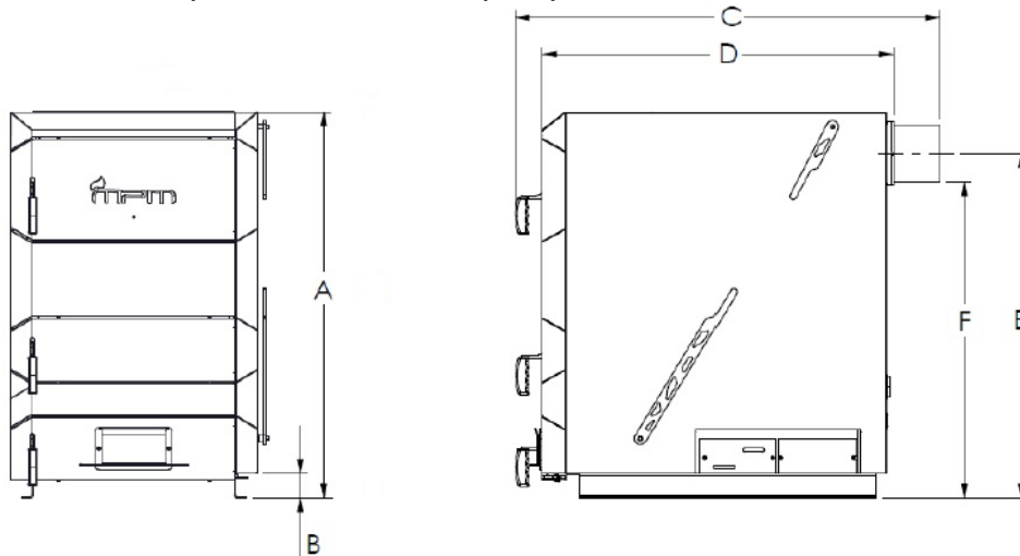
Rysunek 2. Podstawowe wymiary kotła MPM Wood Plus
