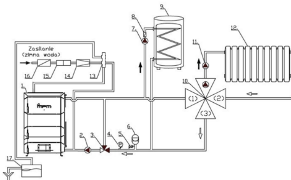
Rysunek 4. Przykładowy schemat podłączenia kotła MPM Wood Plus w układzie zamkniętym.
